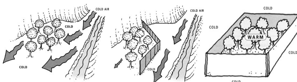
Σχήμα 2.4 Περιγραφή λειτουργίας ανεμόφραξης: α) αφύλακτη καλλιέργεια β) τοποθέτηση ανεμοφρακτών σε μια πλευρά και γ) περιμετρική κάλυψη με ανεμοφράκτες
